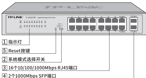
图1-5 TL-SG2218P前面板示意图
