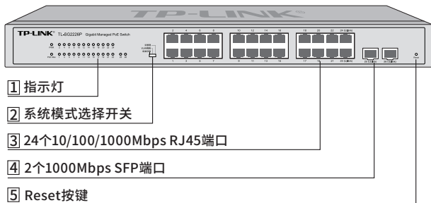
图1-3 TL-SG2226P前面板示意图
